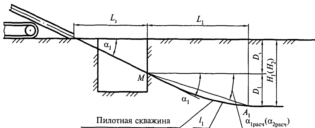
Рисунок Л.1. Основные геометрические параметры трассы
