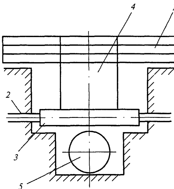
1 - деревянный брус; 2 - кабель; 3 - футляр; 4 - подвеска из скруток проволоки; 5 - прокладываемый газопровод
