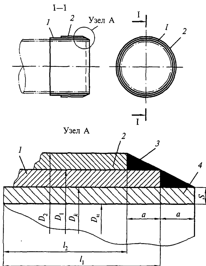
1 - внутреннее кольцо; 2 - наружное кольцо; 3 - наплавка; 4 - прокладываемый футляр
