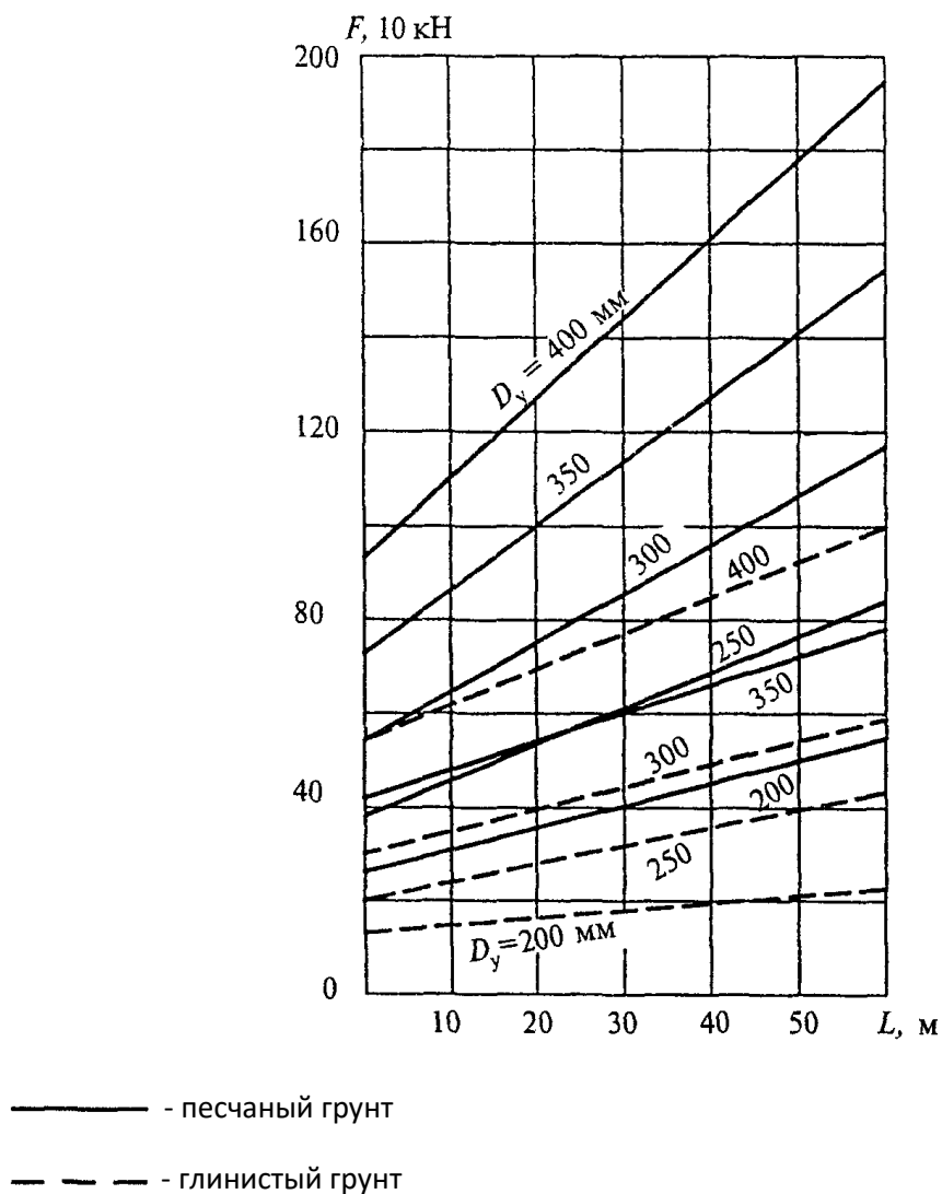
Рисунок 16. Диаграмма зависимости нажимных усилий от длины проходки при прокладке футляров
